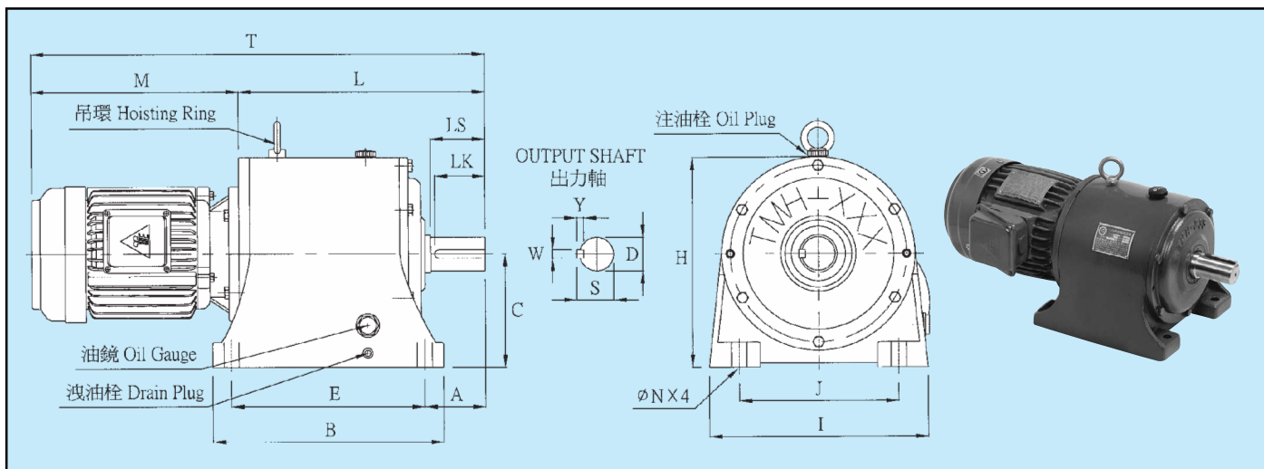
尺寸表 DIMENSION (單位 m/m)
